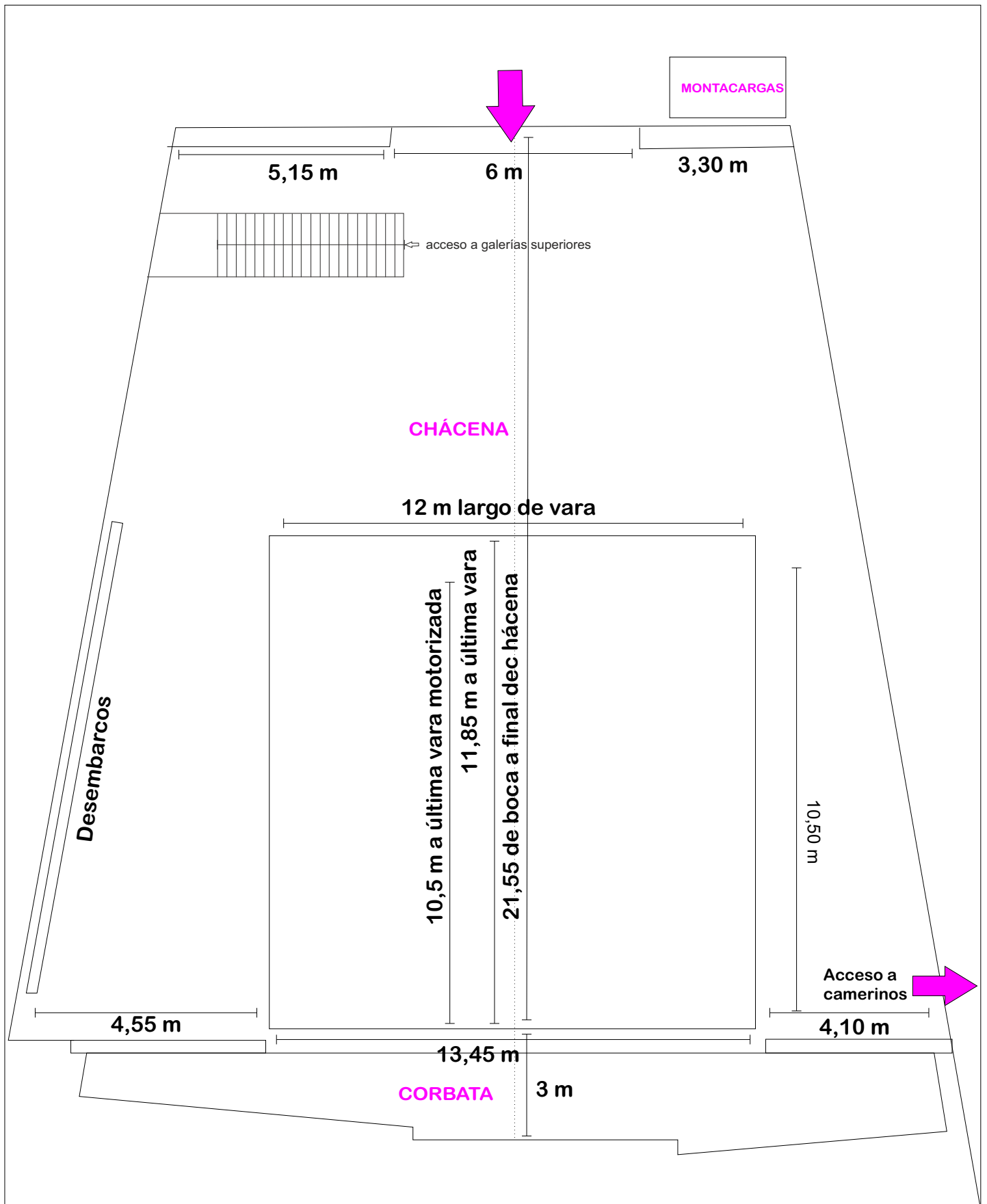
PLANO ESCENARIO TEATRO INFANTA LEONOR COTAS
